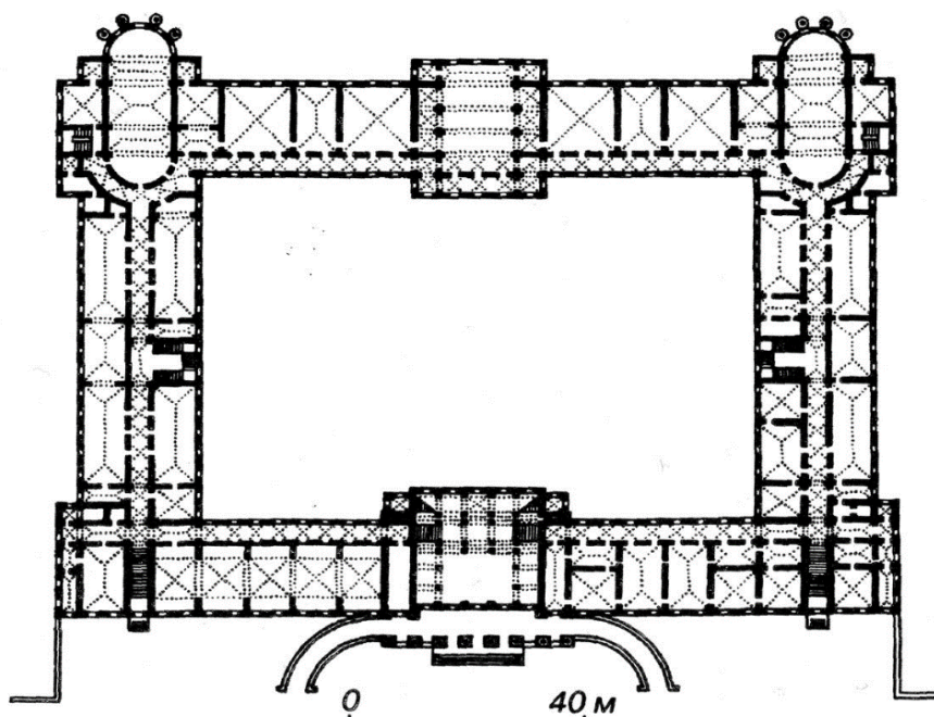
План першого поверху
